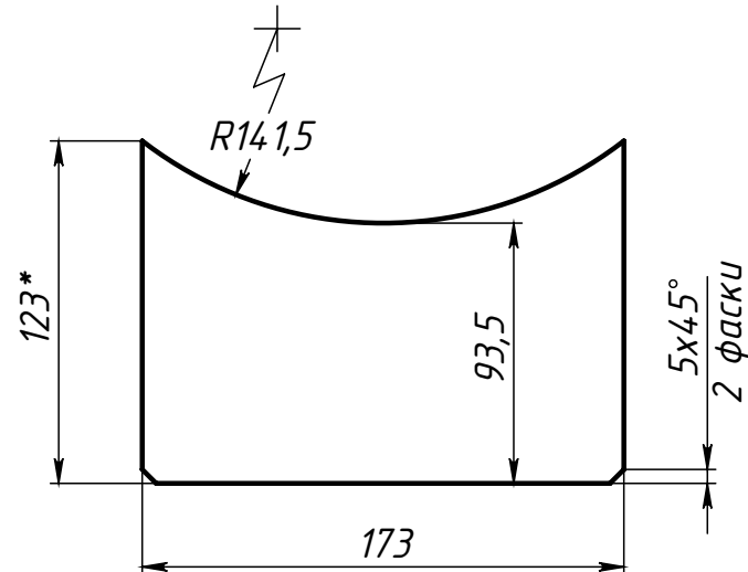
Поз.2 (Ребро)
