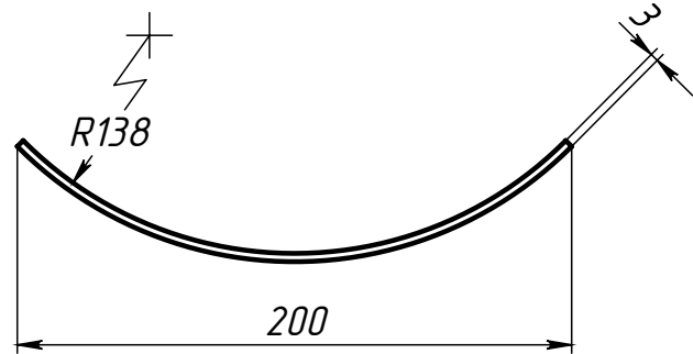
Поз.4 (Подушка)
